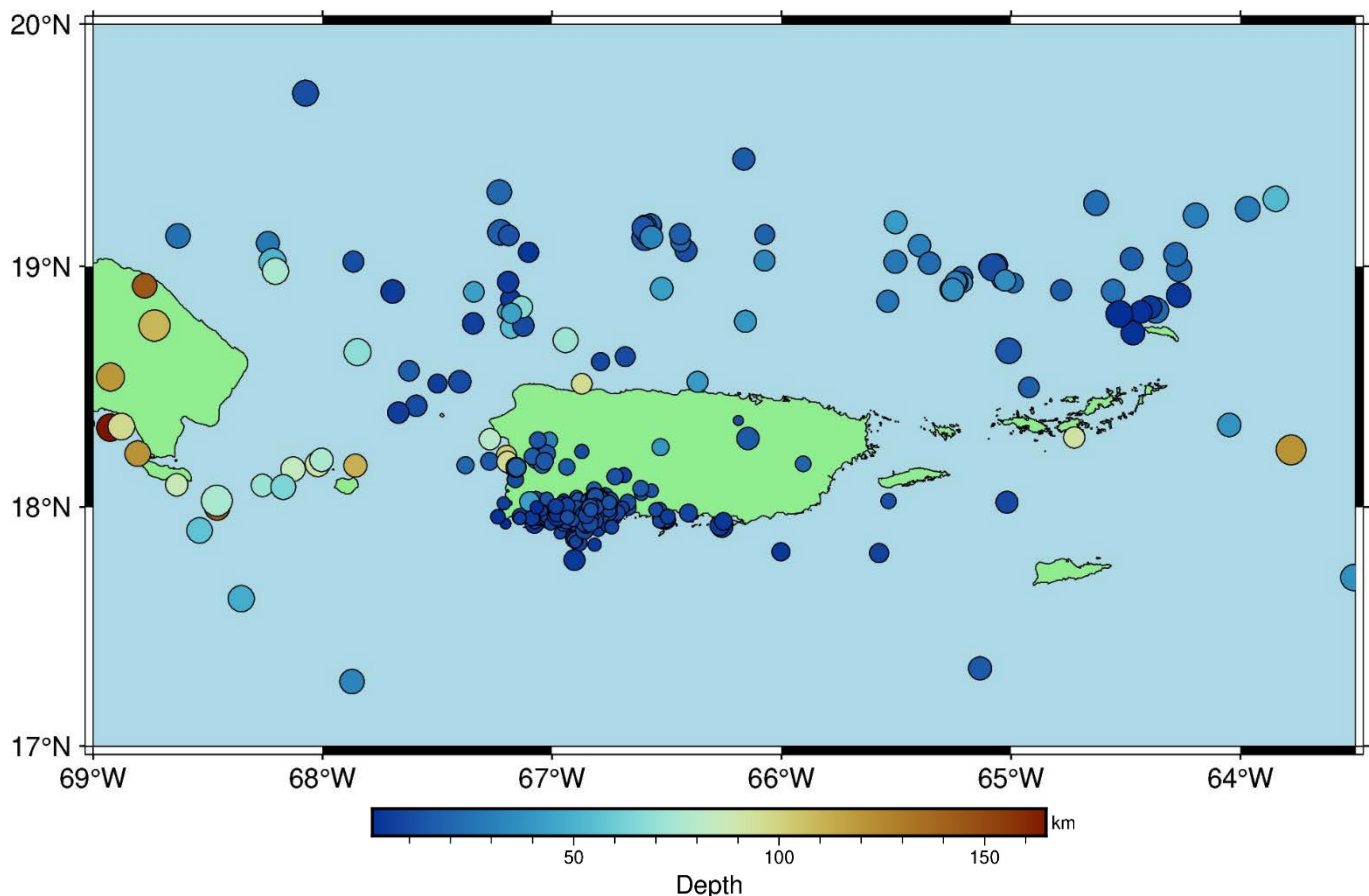
Figura 1. Mapa epicentral de los sismos localizados en la Región de Puerto Rico e Islas Vírgenes por la RSPR para el mes de octubre de 2022 (RSPR-UPRM).
