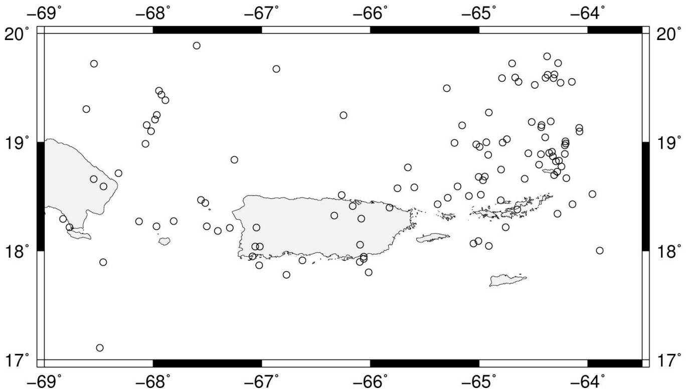
Figura 1. Mapa epicentral de los sismos localizados por la RSPR para el mes de febrero de 2013 (RSPR-UPRM).
